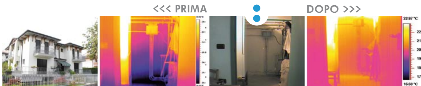
LEGNAGO (VR) - VILLA BIFAMILIARE Impianto installato: n° 1 apparecchio Domodry® LS-R10
